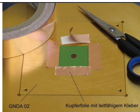
Bild 12 Verkleben des Messsystems für hohe HF - Anforderungen
