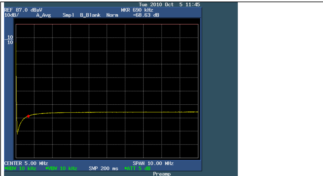
Bild 6 Untere Grenzfrequenz 700kHz des EFM 04
