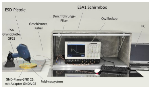
Bild 2 Mess- und Kalibrierplatz für allgemeine Anwendung z.B. Vermessung eines ESD-Generators
