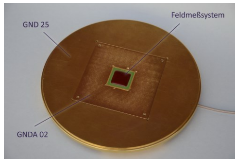
Bild 8 Groundplane GND 25 mit Groundadapter GND A 02 und Feldmesssystem EFM 04 .
