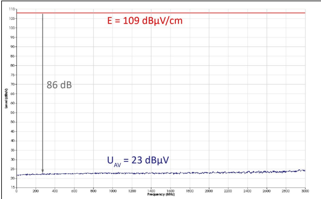
Bild 5 Frequenzgang und Arbeitsweise des EFM 04
